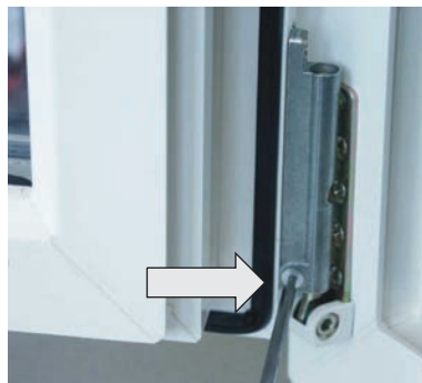
Einstellung der Drehhemmung mit Inbusschlüssel SW2,5 bei Anschlag rechts bei geschlossenem Flügel, bei Anschlag links bei offenem Flügel.
