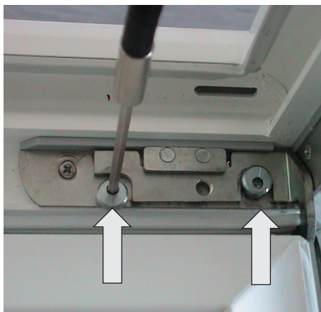
Sicherungsbolzen an beiden Kipplagern mit Inbusschlüssel SW5 um 180° drehen.
