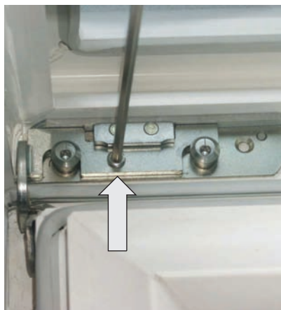
Fixierschraube am Kipplager mit Inbusschlüssel SW4 lösen.
