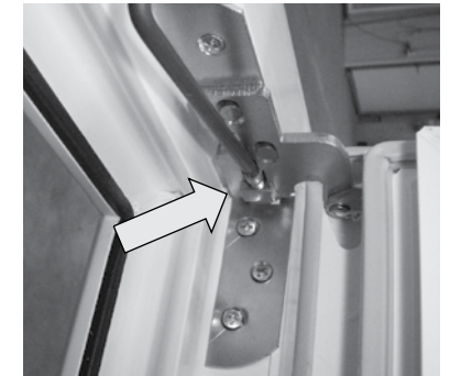
Verstellung bei Schwerlastbeschlag mit Torx T25.
