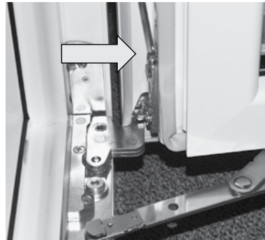
Anheben und Absenken des Flügels mit Inbusschlüssel SW4, bei Schwerlastbeschlag mit Torx T25.
