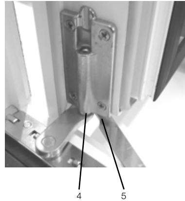
Flügellager KF520
