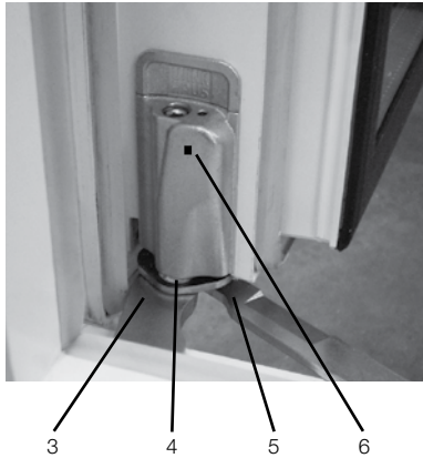
Flügellager KF500
