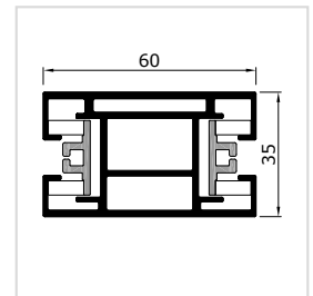
freitragende Kämpferschiene FS ZT60V
