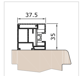
Standard Führungsschiene FS Z37VS
