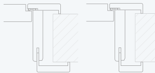
VARIO/INNEN-FB Türblatt gefälzt, öffnet nach innen:
