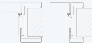
S-DESIGN-FB Türblatt stumpf, öffnet nach außen:
