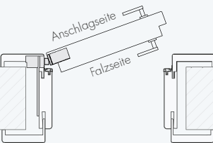
VARIO-FB Türblatt gefälzt, öffnet nach außen:
