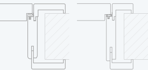
VARIO-FB Türblatt gefälzt, öffnet nach außen:
