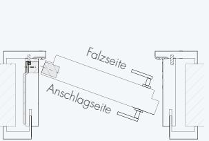
VARIO/INNEN-FB Türblatt gefälzt, öffnet nach innen:
