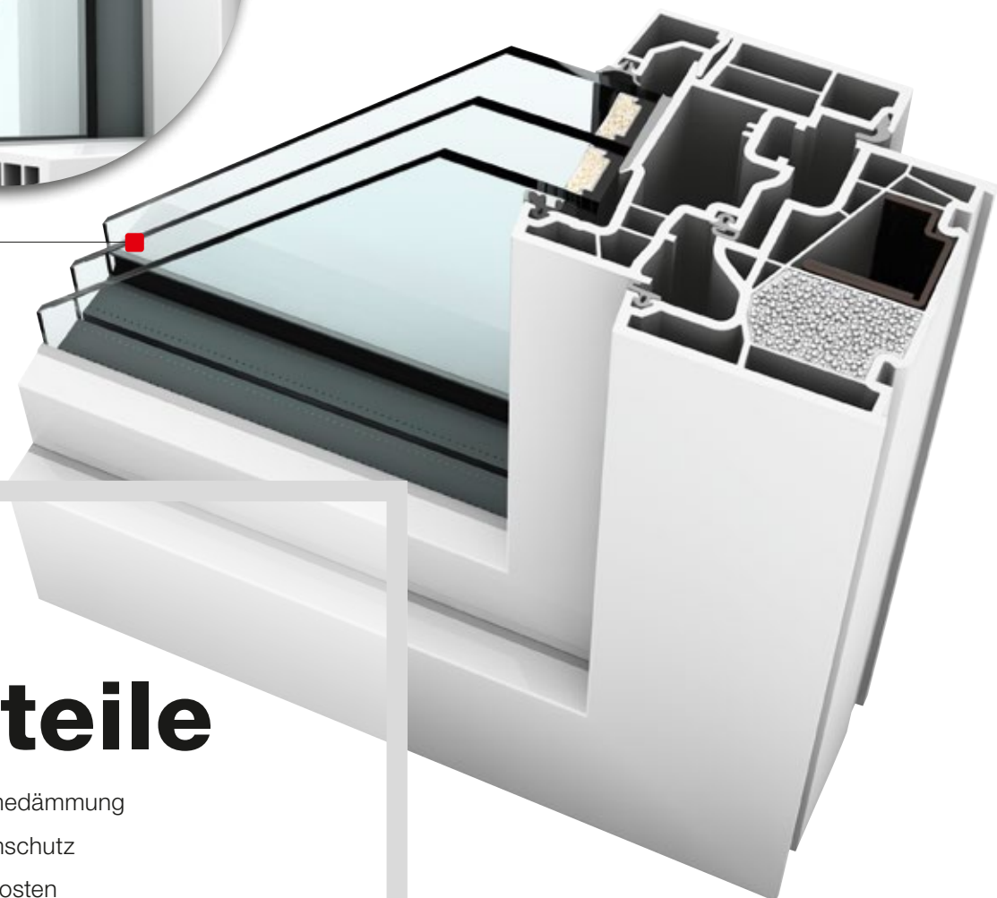
3fach-Verglasung
