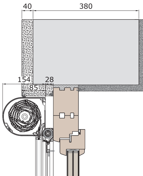
Mit Stockaufdoppelung. VORO BRAVO mit kombiniertem Insektenschutz-Rollo.
